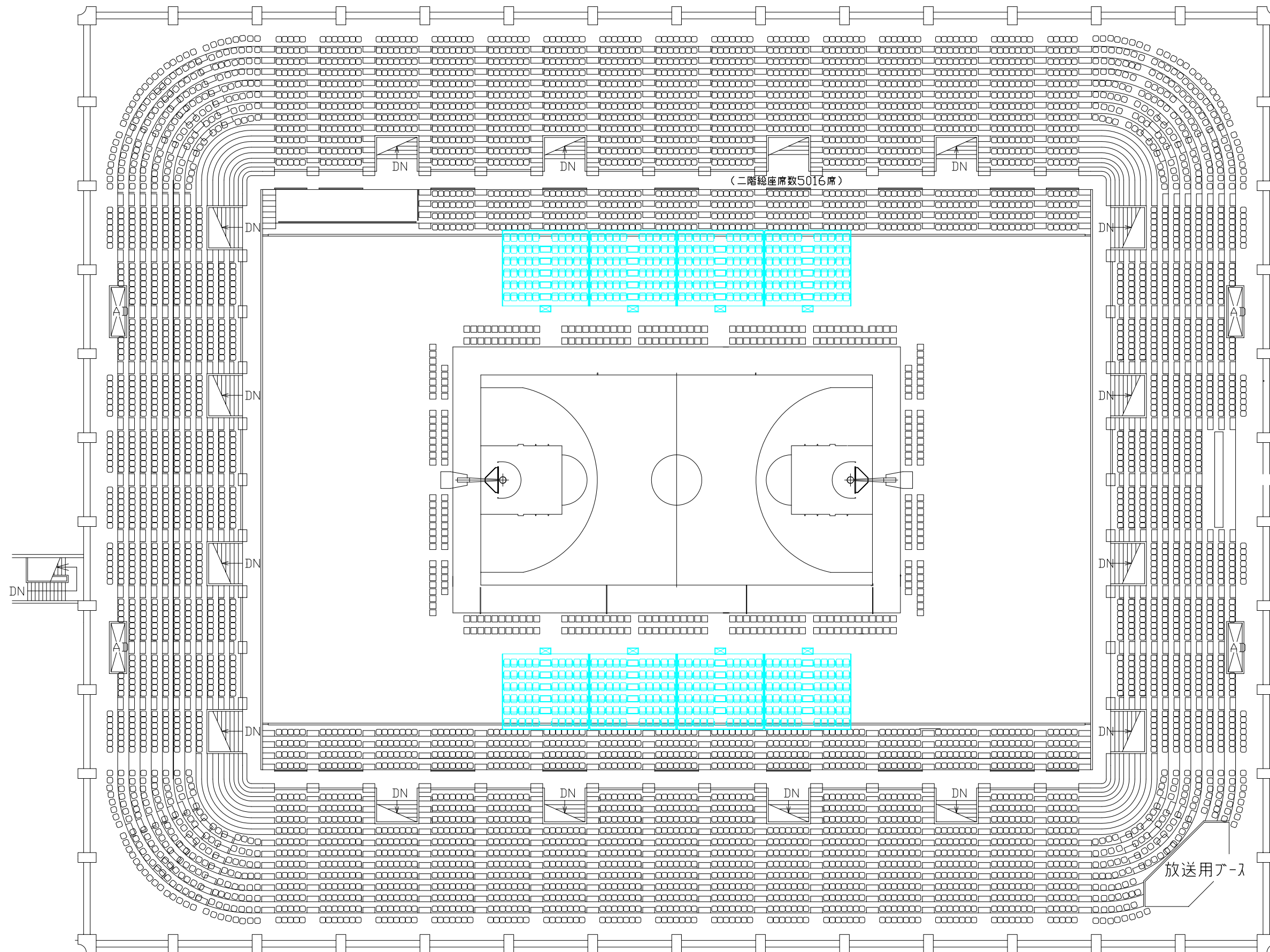
80. 移動式観客席を利用した 競技コート一面の利用例 (バスケットボール、バレーボール、テニス等可)
