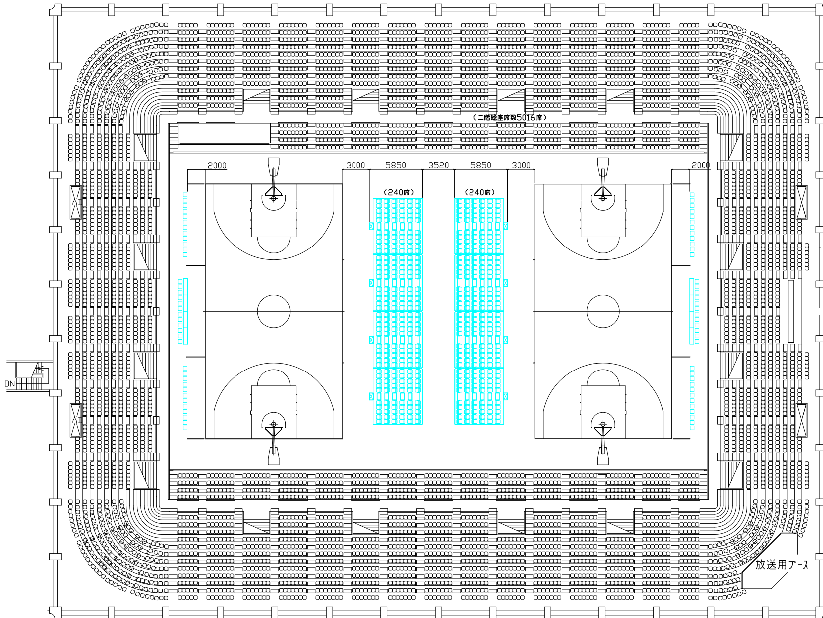
移動式観客席を利用した 競技コート二面の利用例 (バスケットボール、バレーボール、テニス等可)
